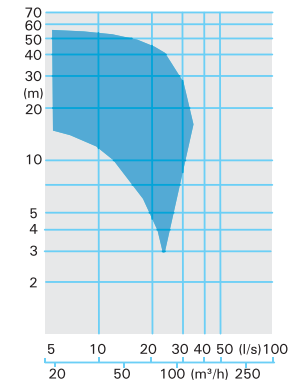
V 23... -2 pole
