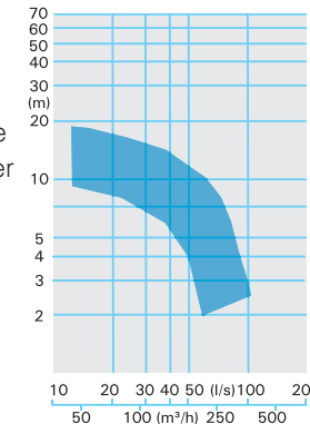
MX 34... -6 pole
