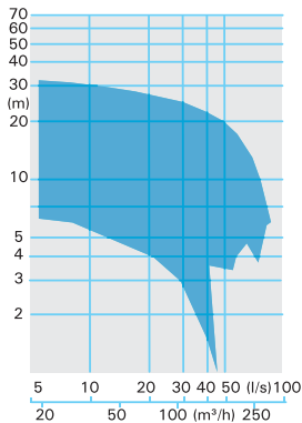
MX 24... -4 pole
