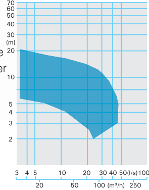
MX 13... -4 pole
