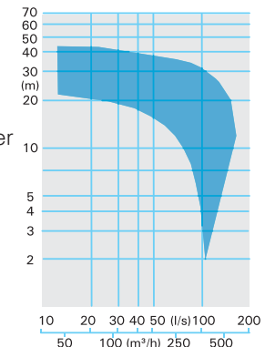
K 33... -4 pole
