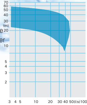
MX 13... -2 pole
