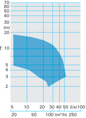
MX 23... -4 pole
