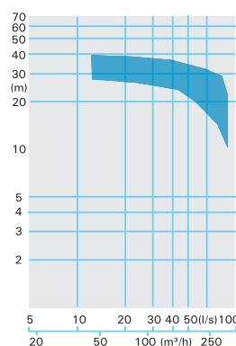
VX 34... -4 pole
