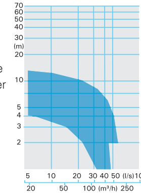
MX 24... -6 pole
