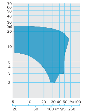
VX 24... -4 pole
