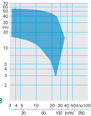
V 13... -2 pole
