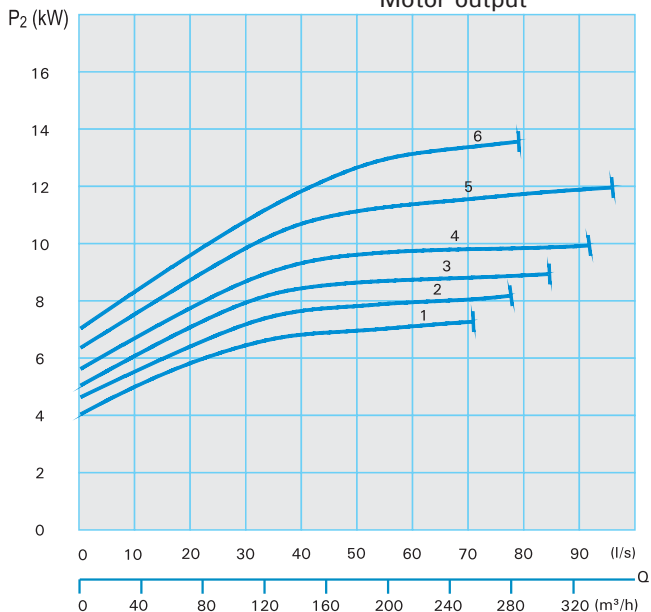
Motor output
