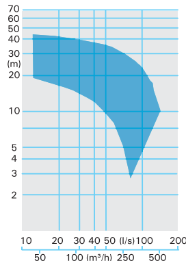
MX 34... -4 pole
